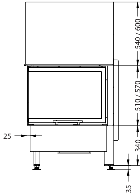
Vorderansicht M~1:20
