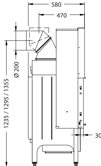
Seitenansicht M~1:20
