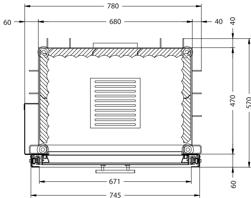
Horizontalschnitt M~1:10
