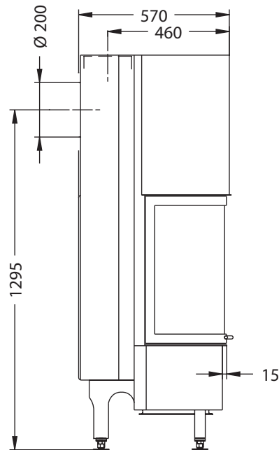
Seitenansicht M~1:20
