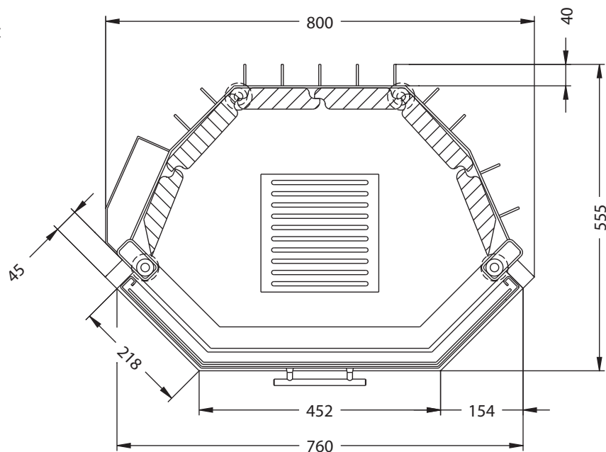
Horizontalschnitt M~1:10
